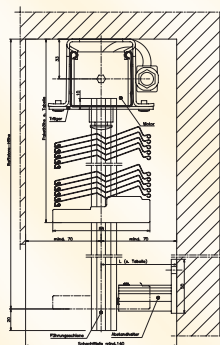
EL 88 AS Z-Lamelle 88mm mit Motor und Führungsschienen
