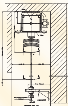
EL 50 A Lamellenbreite 50mm mit Motor und Seilführung
