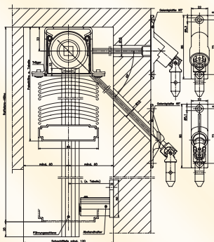
K 60/80 AS Lamellenbreite 60/80mm mit Knickkurbel und Schienenführung, optional mit Motorbedienung
